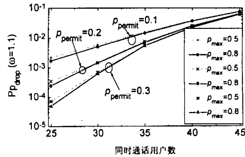
图 5 VP-PRMA 方法中不同 p_{\max} 下的情况
