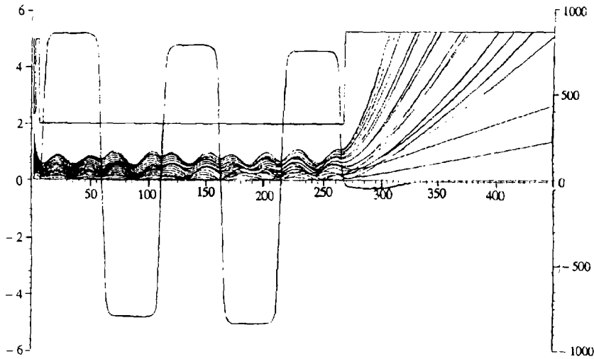
图 6 电子光学系统的电子轨迹
