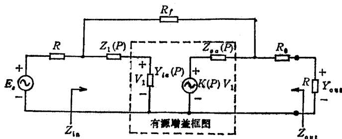
图 1 基本反馈放大器
