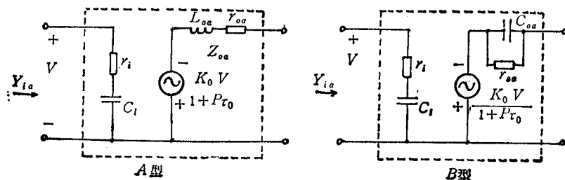
图4 增益框图的模型
