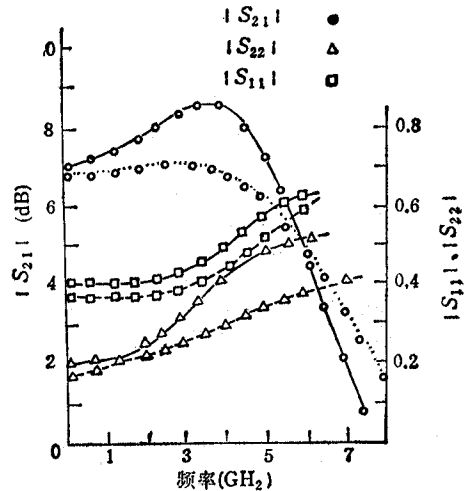
图 7 原始响应和优化响应曲线
