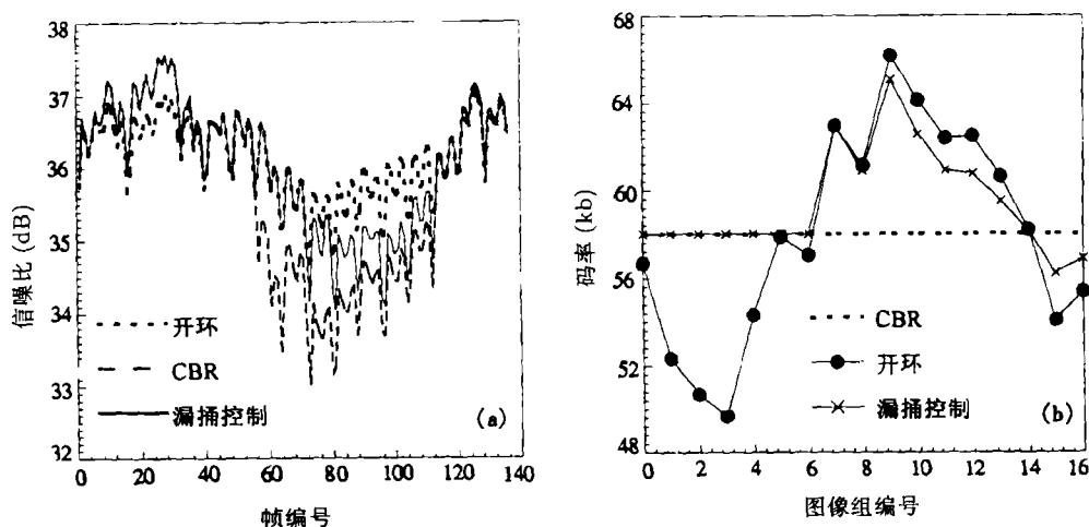
图 5 “Miss America” 序列分别在开环、不变比特率和漏桶控制下的 (a) 恢复图像的信噪比较; (b) 码率比较
