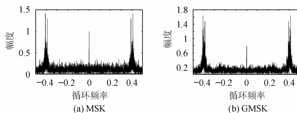
图7 -10\text{dB} 下 MSK 和 GMSK 信号 f=0 的 \alpha 截面谱
