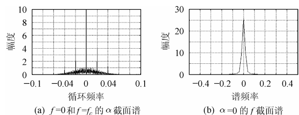
图6 h=1, T=50s 的基带循环谱
