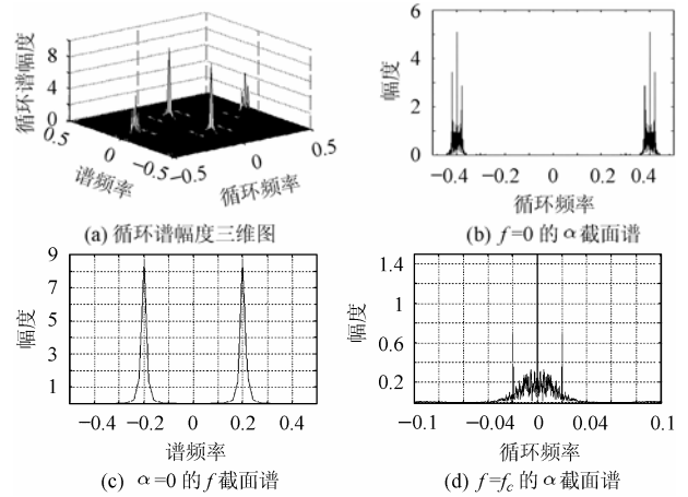
图 3 调制指数为 h=1 , 脉冲长度 L=2 时 CPM 信号的循环谱
