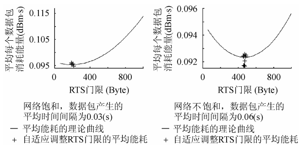
图1 RTS门限调整效果
