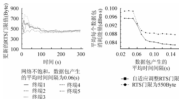
图3 RTS门限更新过程
