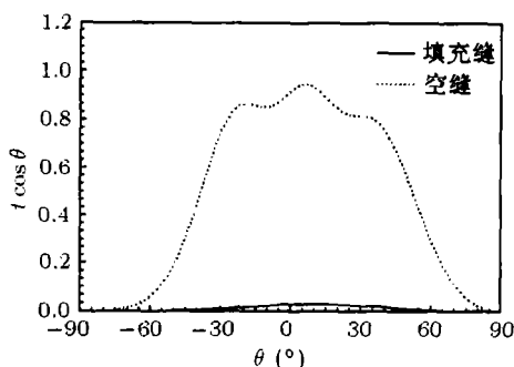
图 8 传输系数随入射角变化曲线
