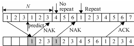
图 2 预重传 GBN-ARQ 方案 1
