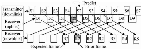
图 1 预重传 GBN-ARQ 方案
