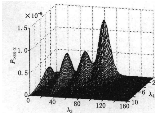
图 2 3 型和 4 型阻塞 2 型的概率 P_{>34:2|T}(\lambda_3, \lambda_4)
