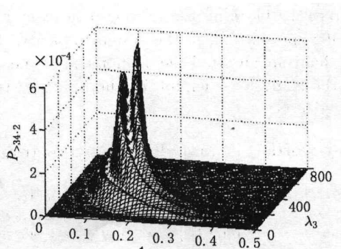
图 3 3 型和 4 型阻塞 2 型的概率 P_{>34:2|T}(\lambda_3, t)
