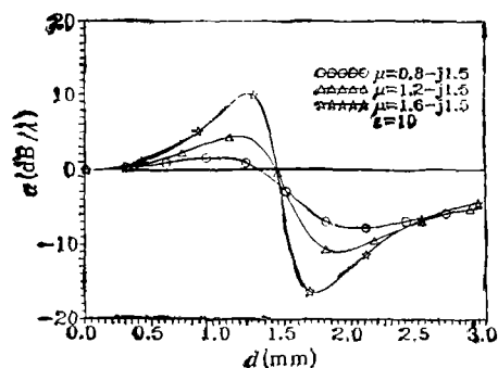
图 5 \mu 实部对 \alpha 的影响
