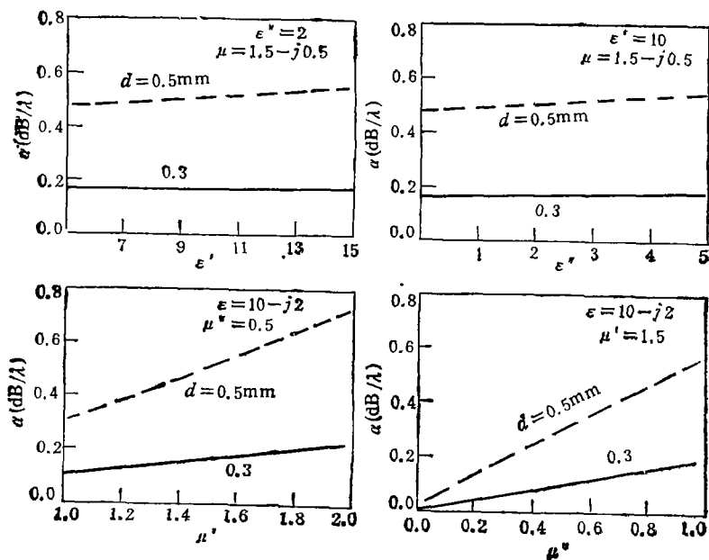
图 7 d = 0.3\text{mm}, d = 0.5\text{mm} 时, \alpha 与 \varepsilon, \mu 的实部、虚部的关系曲线
