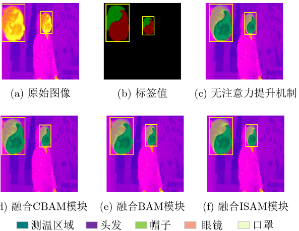
图 4 红外空间注意力模块目标检测阶段有效性测试
