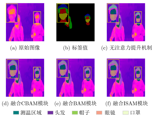
图5 红外空间注意力模块目标分割阶段有效性测试
