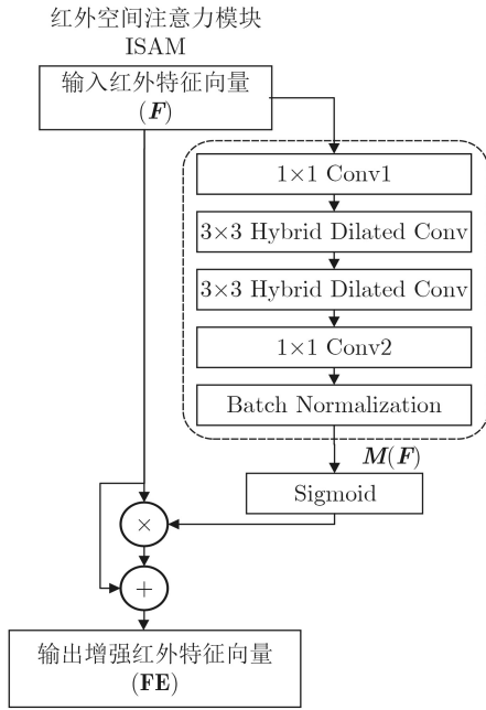
图3 红外空间注意力模块结构
