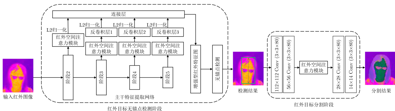
图2 用于红外热成像温度测量区域分割的无锚点实例分割网络结构
