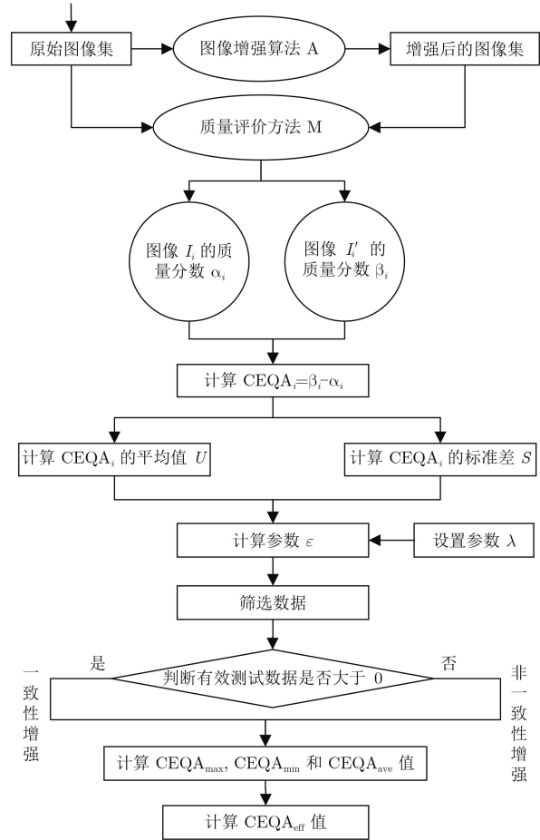
图6 CEQA准则的流程图
