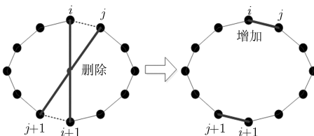
图 3 2-opt 算法示意图
