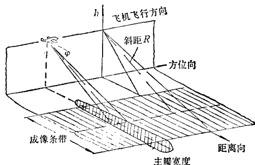
图 1 机载侧视 SAR 工作几何关系示意图
