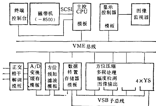
图 3 采用专用高速运算模板的成像器结构示意图
