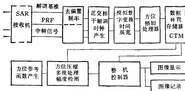
图 2 机载 SAR 实时数字成像处理器原理框图
